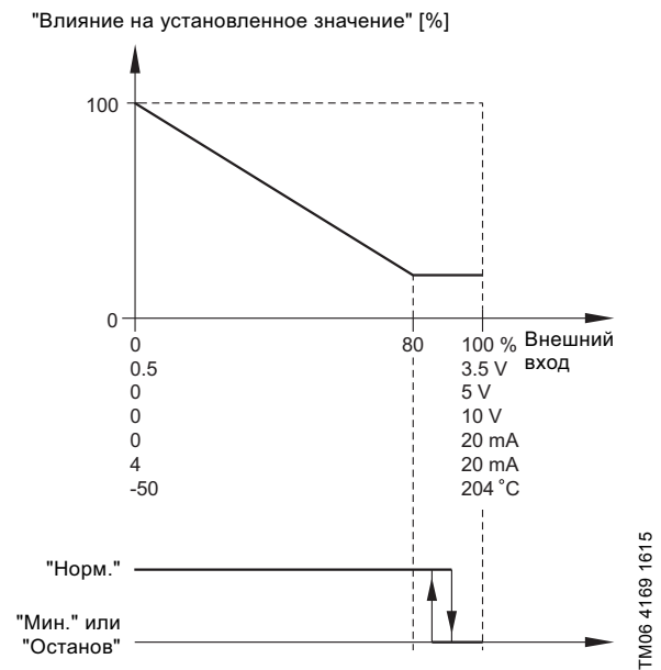
Рис. 77 "Обратная зависимость с остановом" и "Обратная зависимость с минимальной характеристикой."
