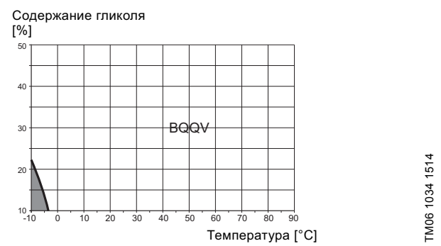
Рис. 6 Рабочий диапазон торцевых уплотнений из FKM
